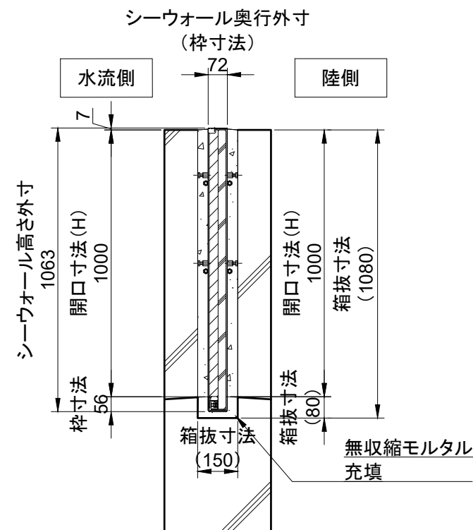
A-A' 矢視図 (S = 1 : 20)
