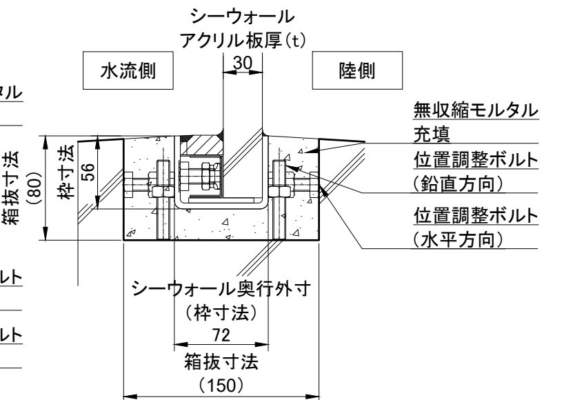
標準部断面詳細図 (S = 1 : 20)
