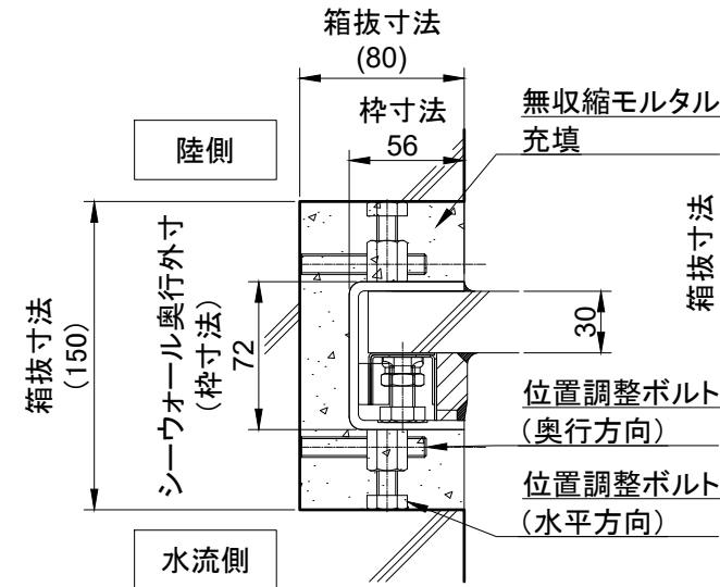
A-A' 矢視図 (S = 1 : 20)
