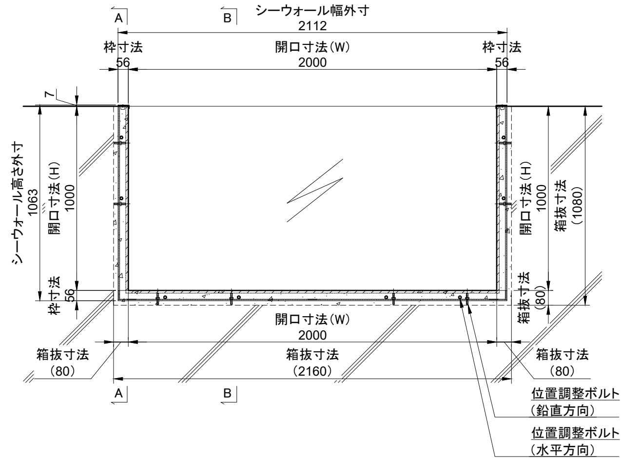
正面図 (S = 1 : 20)
