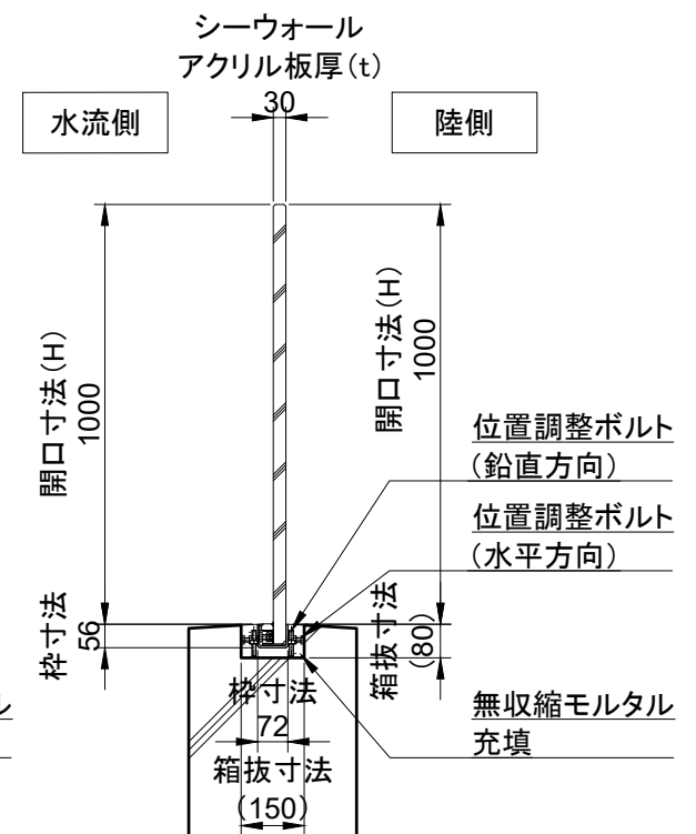
B-B' 矢視図 (S = 1 : 20)
