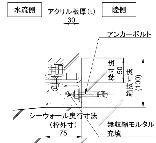
断面図 (S = 1 : 20)
