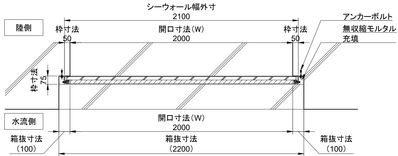
正面図 (S = 1 : 20)
