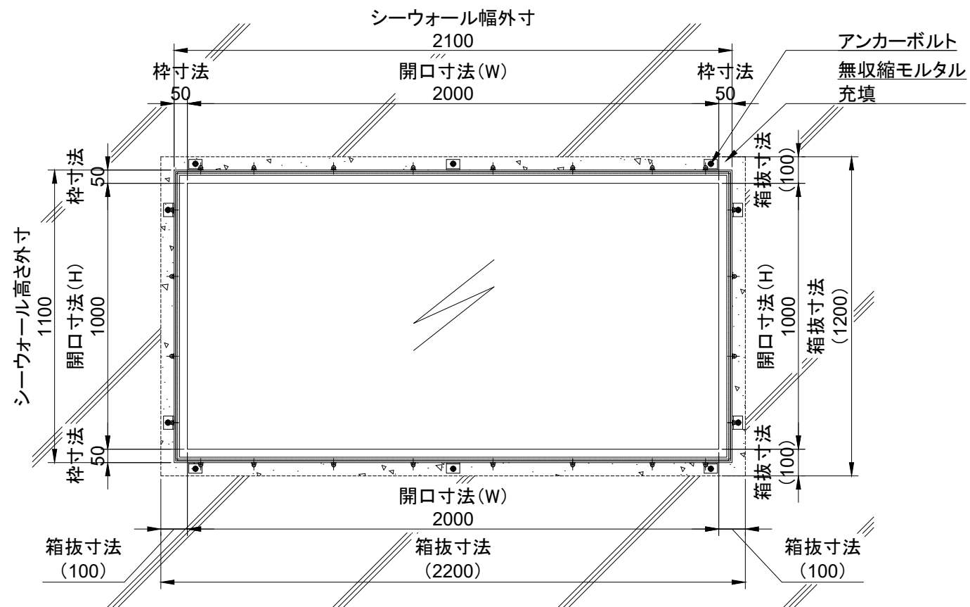
正面図 (S = 1 : 20)
