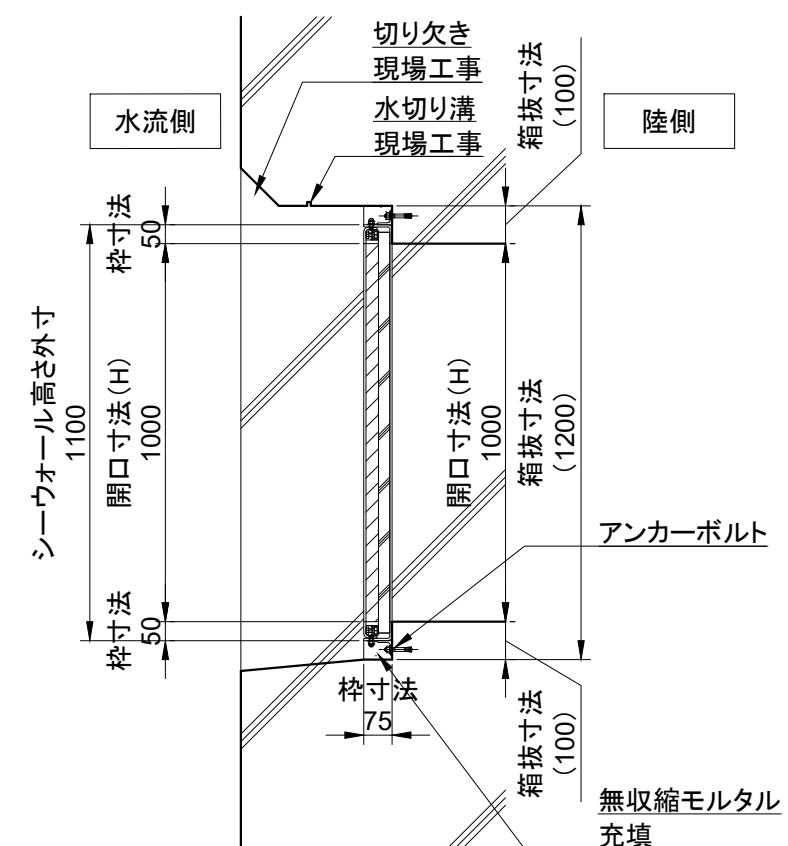
断面図 (S = 1 : 20)
