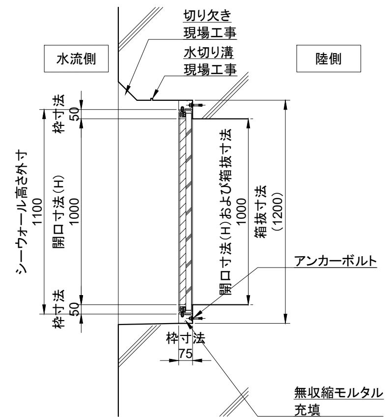
断面図 ( S = 1 : 20 )
