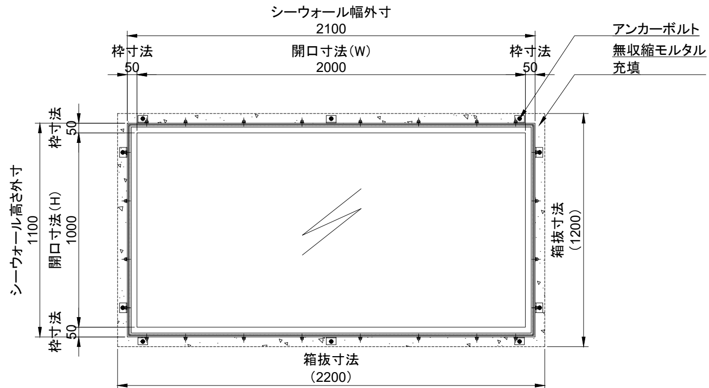
正面図 ( S = 1 : 20 )
